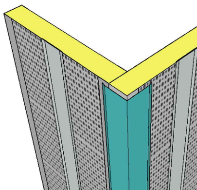
PERFIL ESQUINA CON IP50/05
