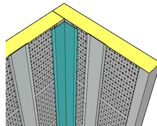
PERFIL RINCON CON IP50/04
