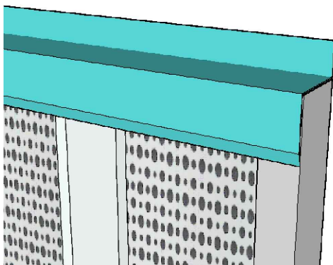
PERFIL IP50/01 - ZONA SUPERIOR
