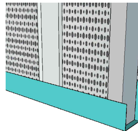
PERFIL IP50/02 - ZONA INFERIOR
