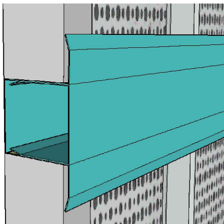
PERFIL IP50/03 - ZONA INTERMEDIA
